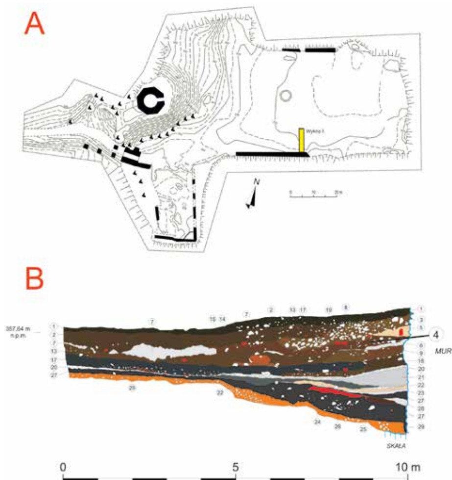
Ryc. 2. Plan zamku ojcowskiego z lokalizacją wykopu I (A) i profil wschodni wykopu I z wyszczególnieniem warstwy 4 (B). Rys. Michał Wojenka
